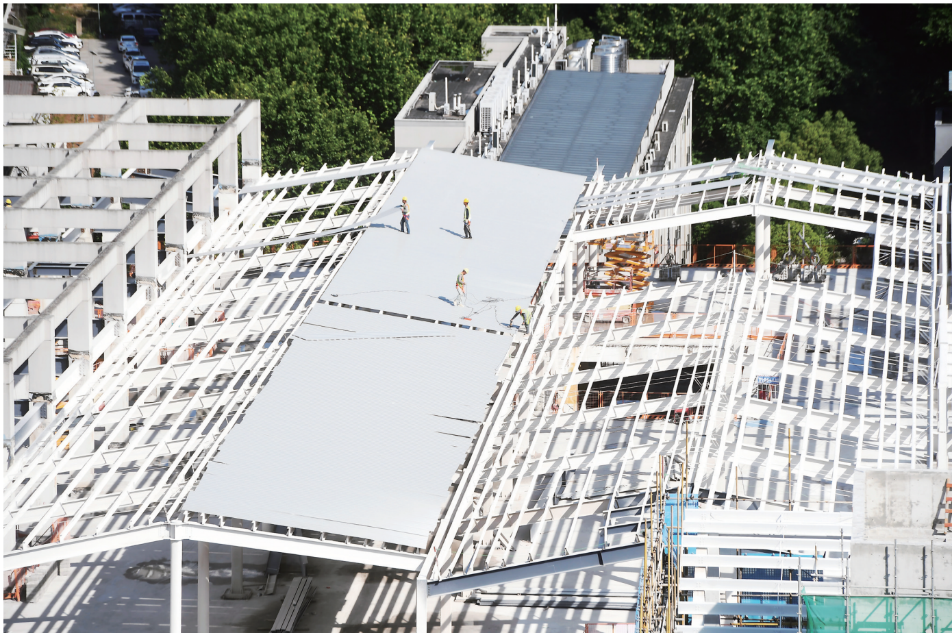
正在建设的广埠屯·锦鲤。
